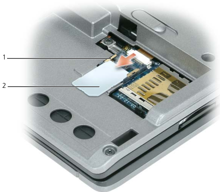
1 SIM カードスロットの金属製タブ (2) 2 角が欠けている SIM カード
